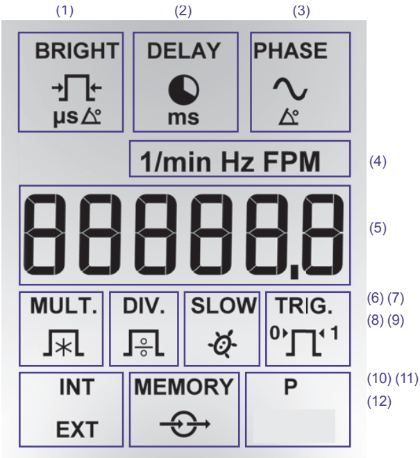
Fig. 2 - Display
